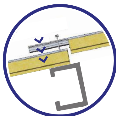
DETALLE TRASLAPE
